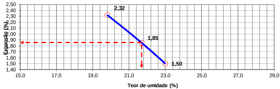
CURVA DA EXPANSÃO
