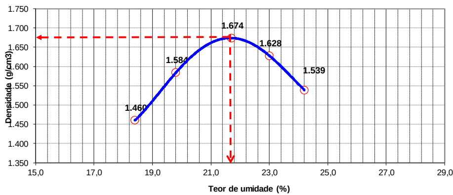
CURVA DA COMPACTAÇÃO
