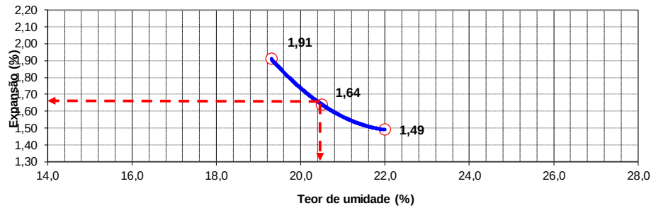
CURVA DA EXPANSÃO
