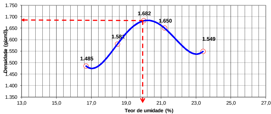
CURVA DA COMPACTAÇÃO
